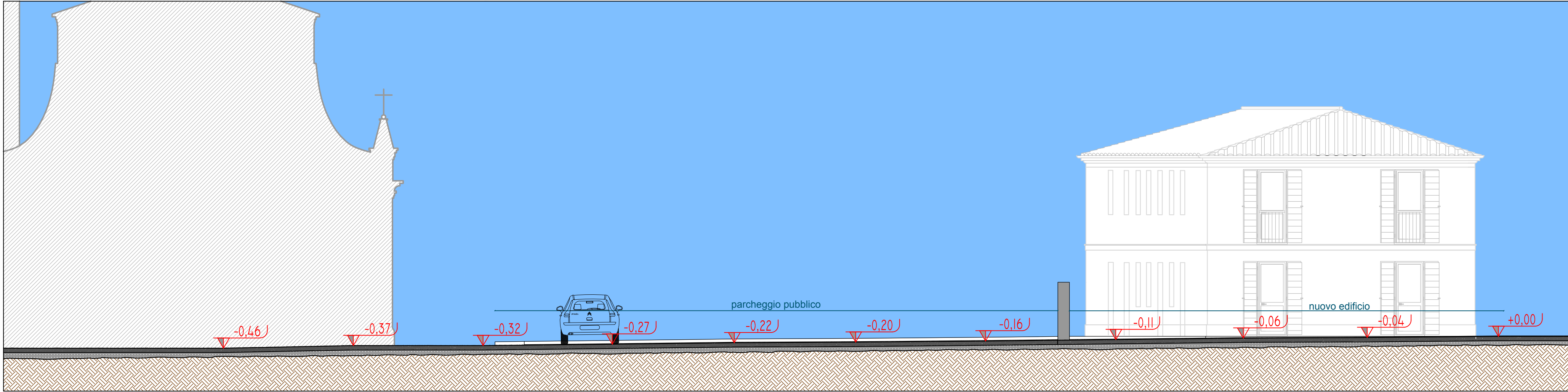
SEZIONE STRADALE BB' SCALA 1:100
