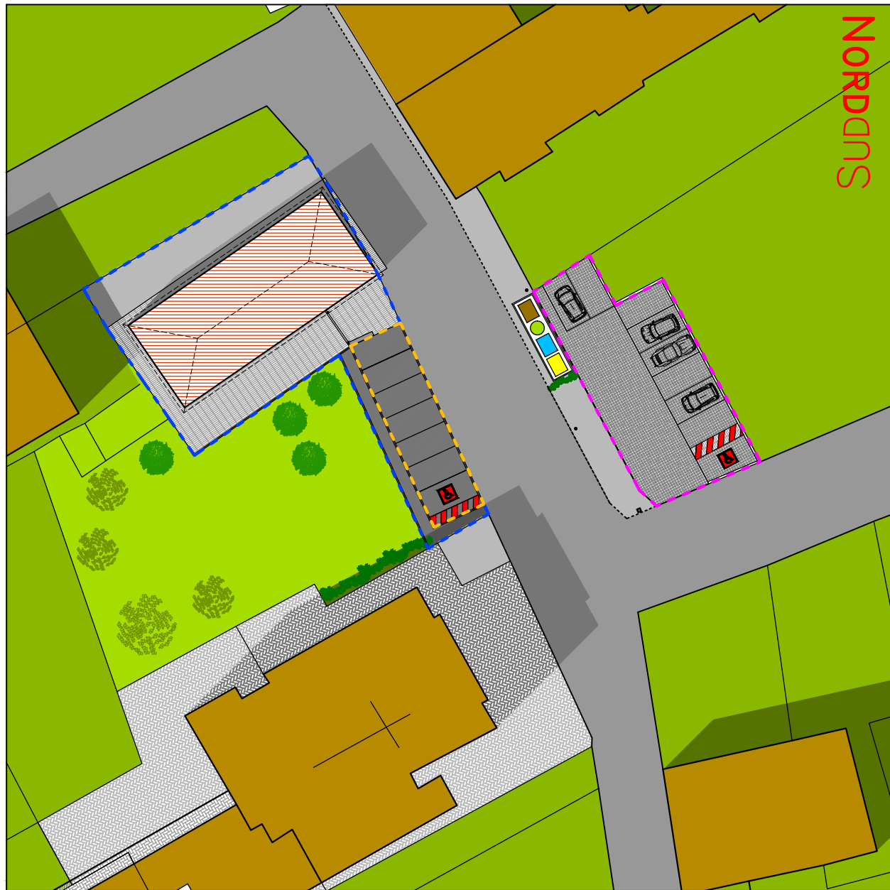
PLANIVOLUMETRICO SCALA 1:500
