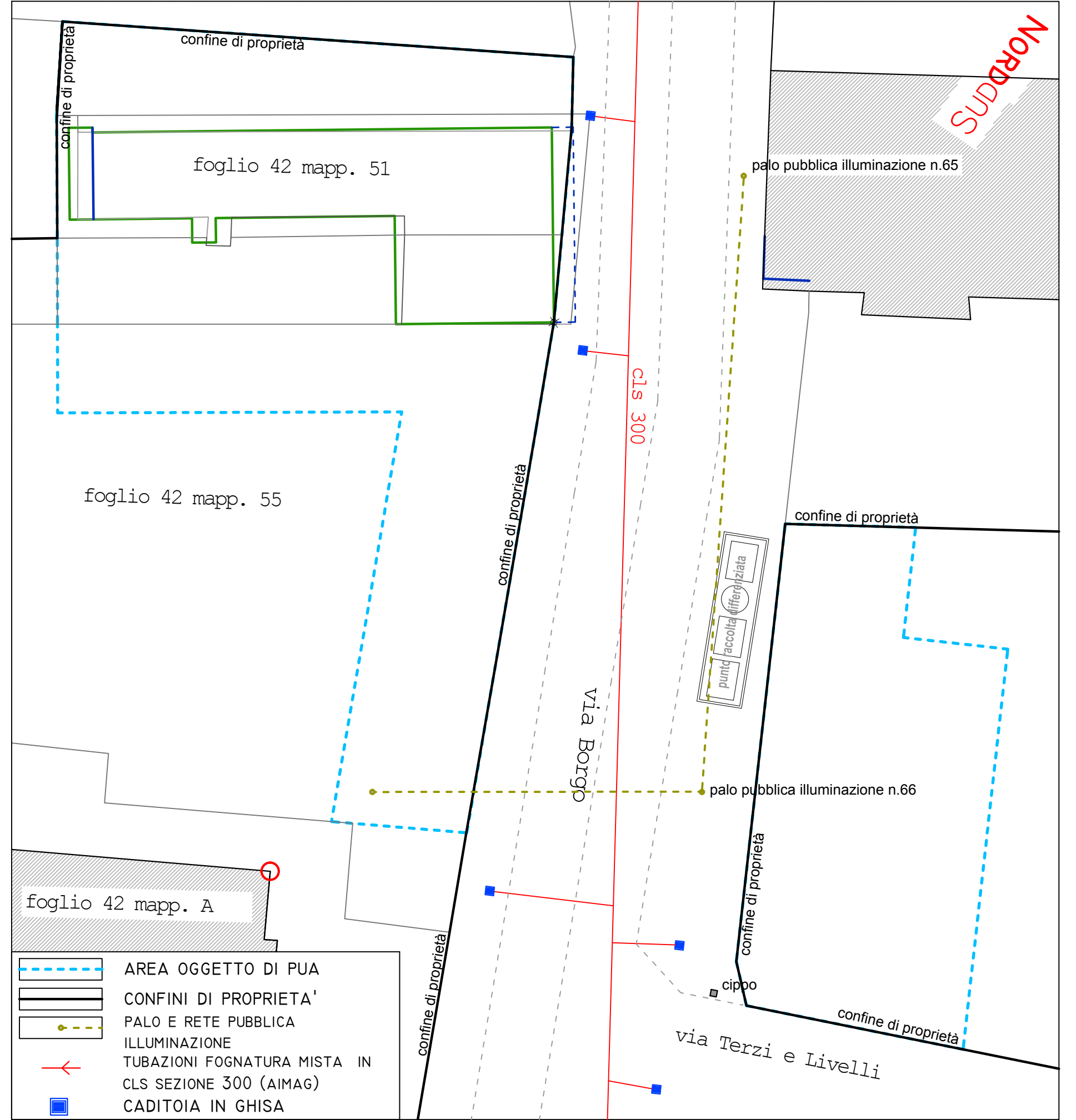
IMPIANTO FOGNARIO E PUBBLICA ILLUMINAZIONE SCALA 1:200
